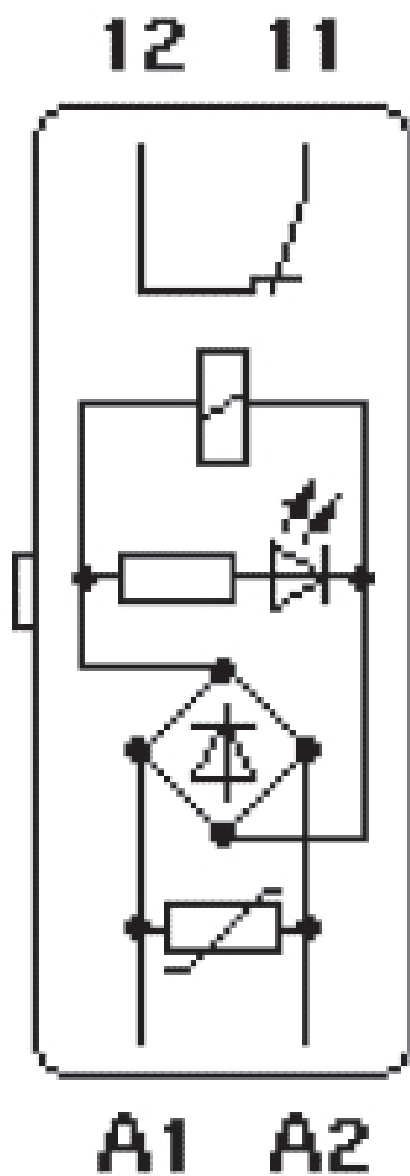
schakelschema
