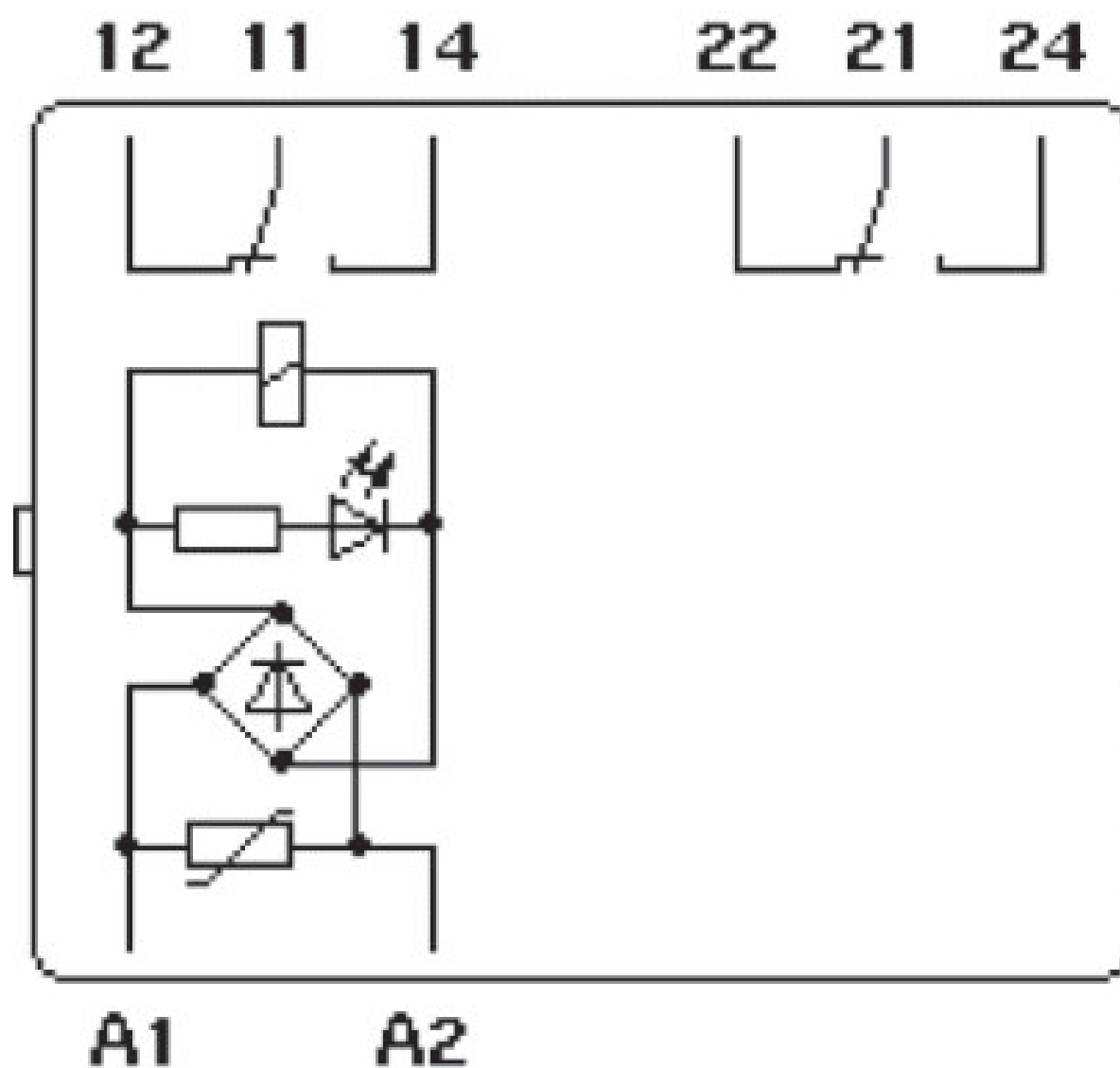
schakelschema
