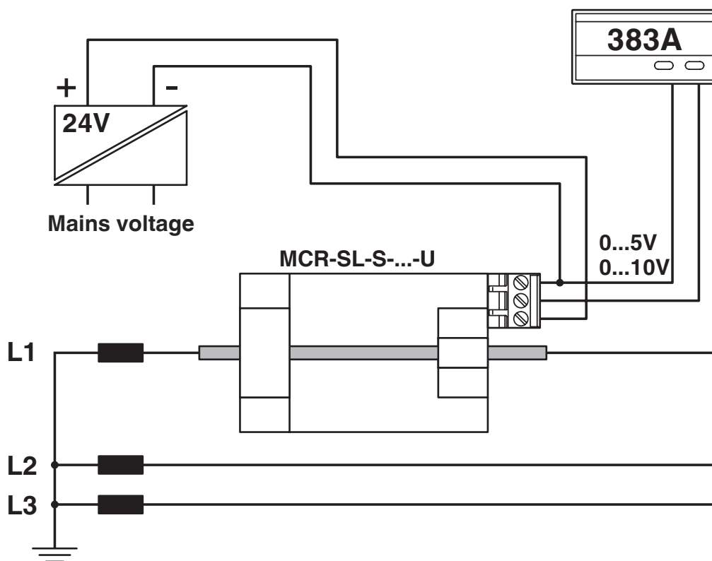
applicatietekening
