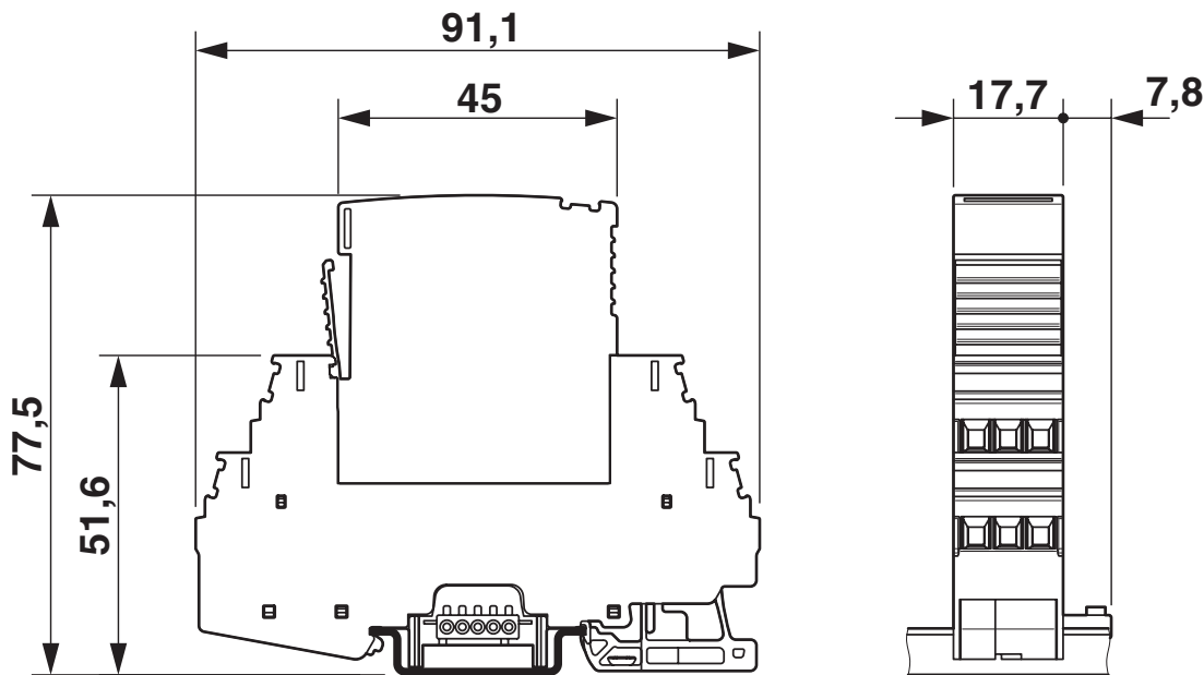
Maatschets
