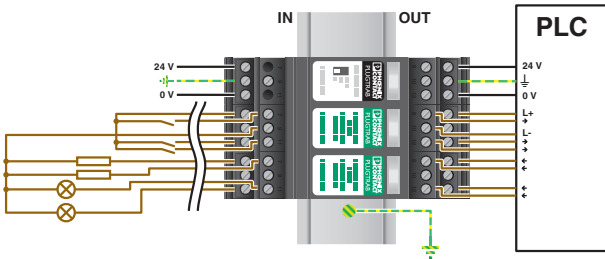
applicatietekening
