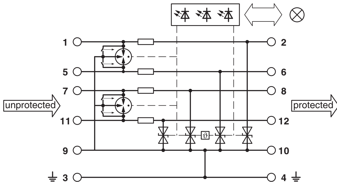
schakelschema
