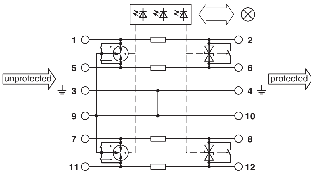
schakelschema
