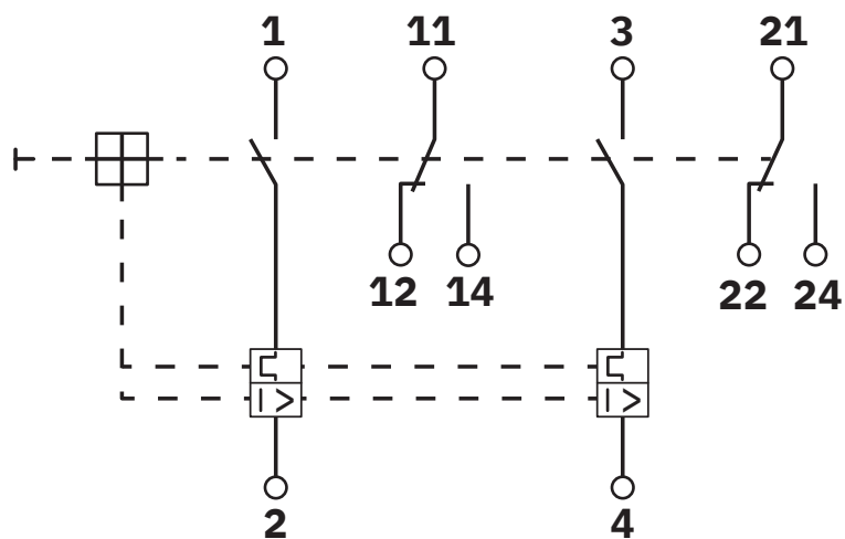
schakelschema
