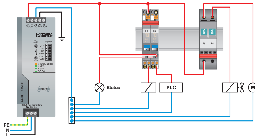
applicatietekening
