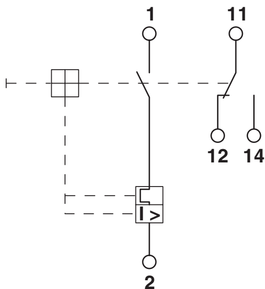
schakelschema
