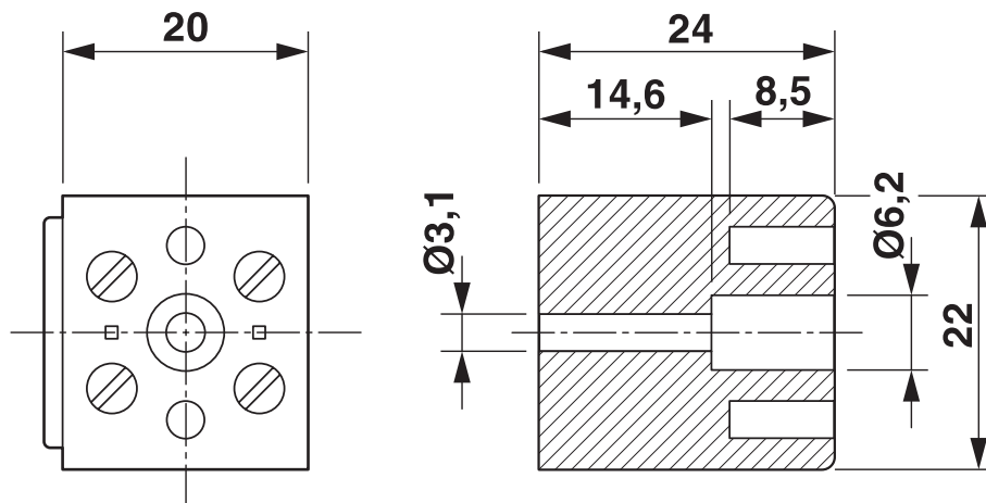
Maatschets
