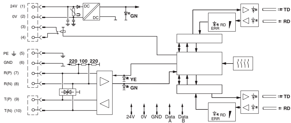
blokschema
