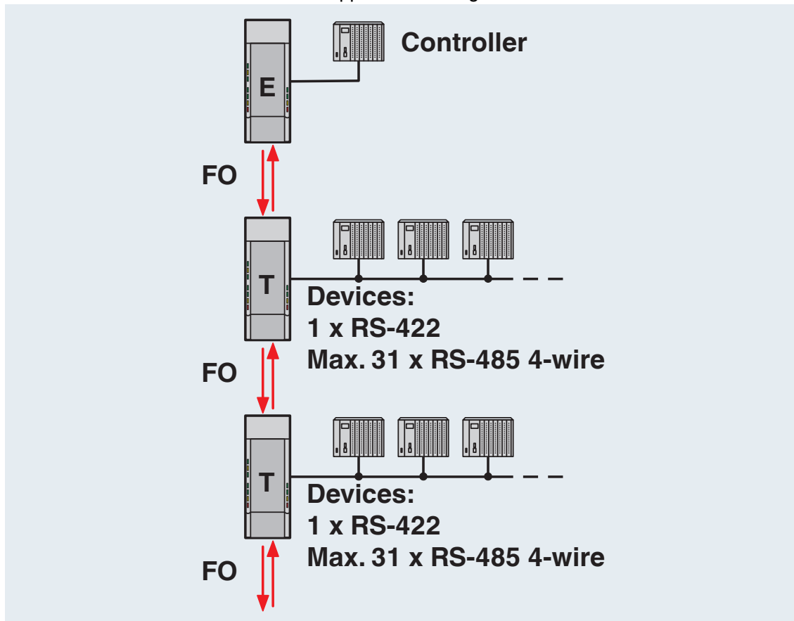
Controller-device-lijnstructuur
