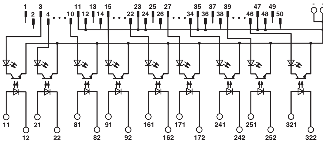
aansluitschema
