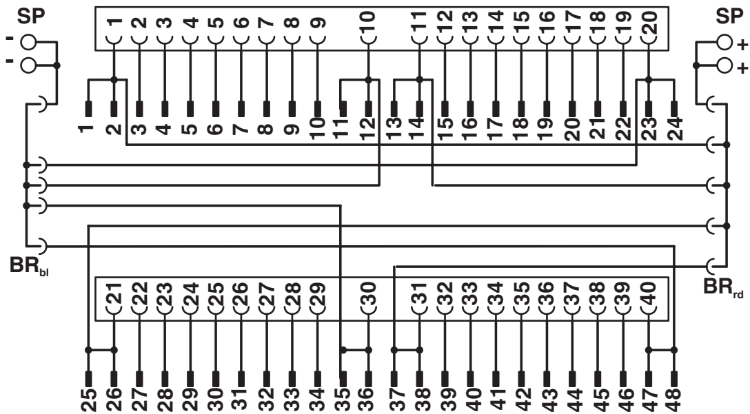
schakelschema
