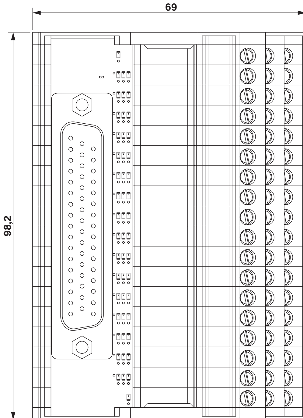
Maatschets
