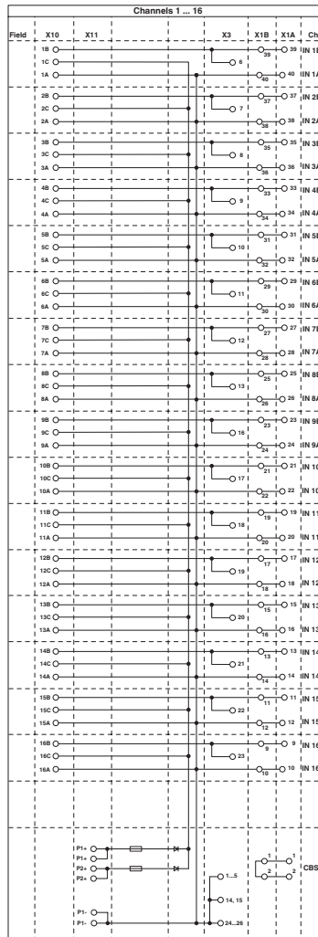
schakelschema
