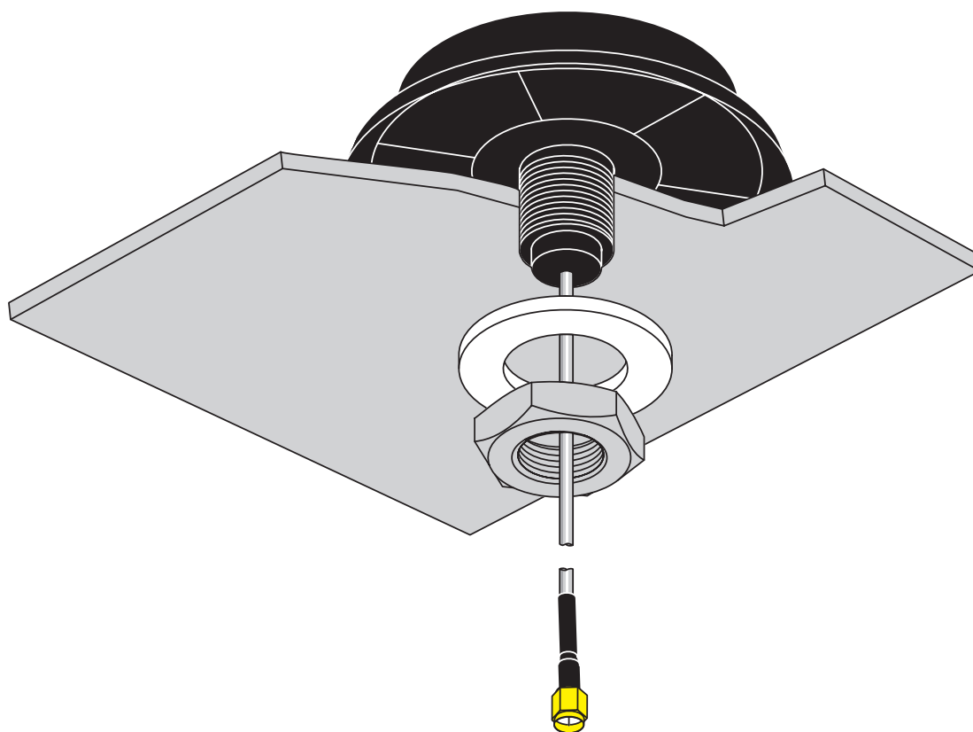
schematekening
