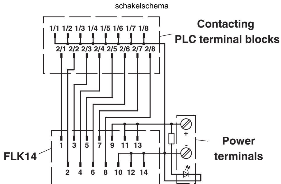
Aansluitschema PLC-V8/FLK14/IN/M
