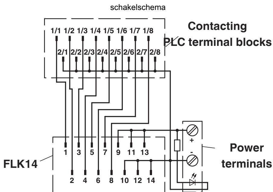
Aansluitschema PLC-V8L/FLK14/OUT
