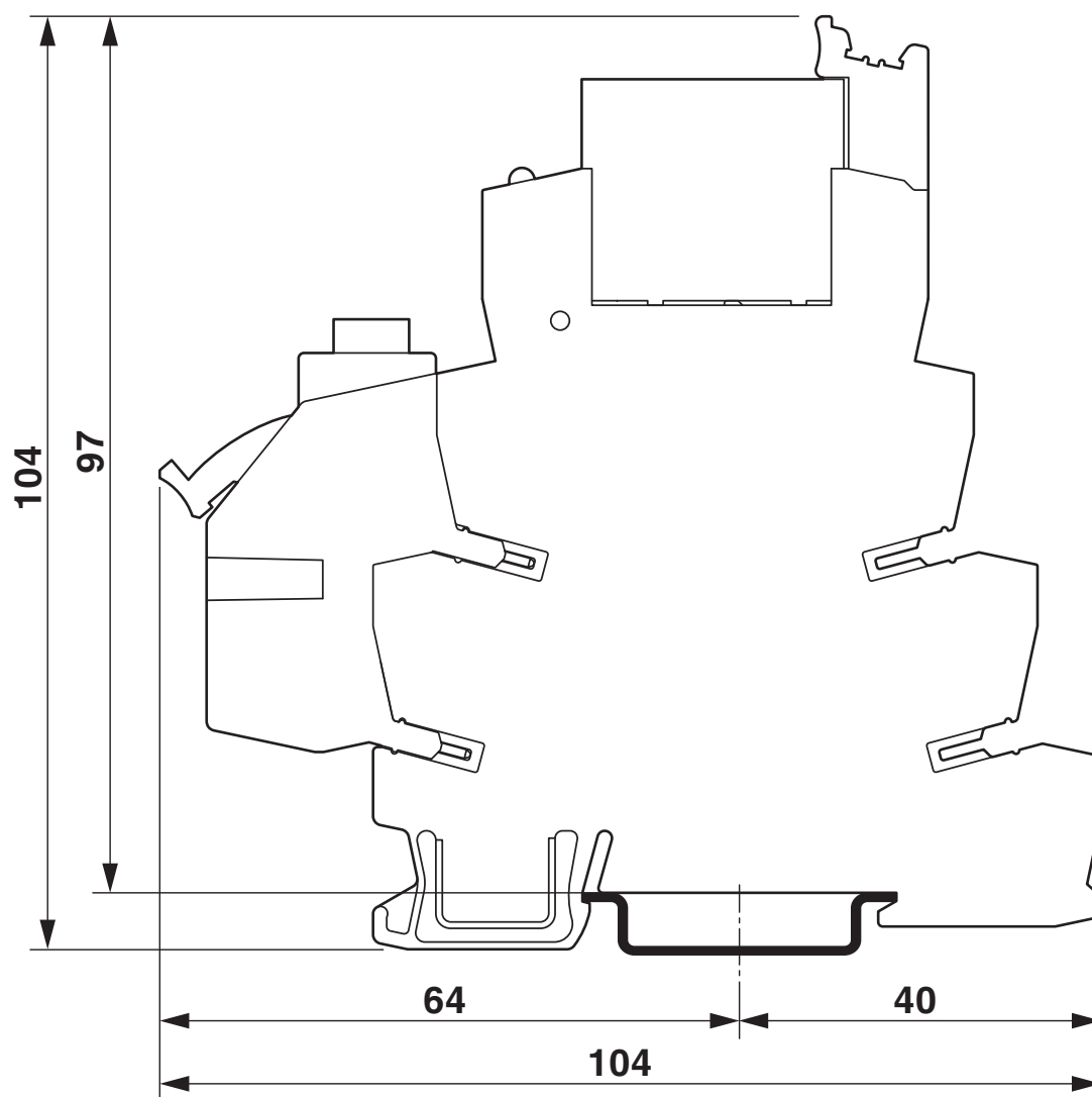
Maatschets
