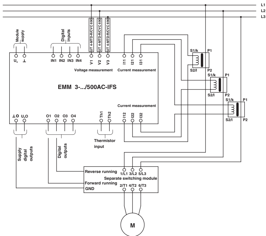
aansluitschema
