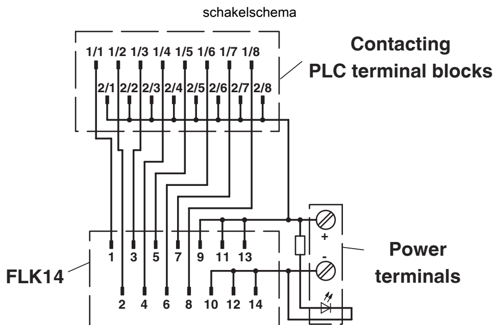
Aansluitschema PLC-V8/FLK14/IN
