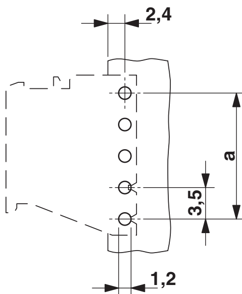
boorsjabloon/soldeerpadgeometrie
