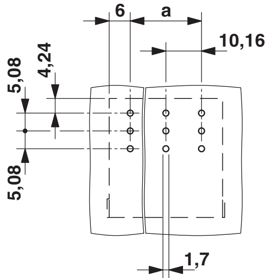
boorsjabloon/soldeerpadgeometrie
