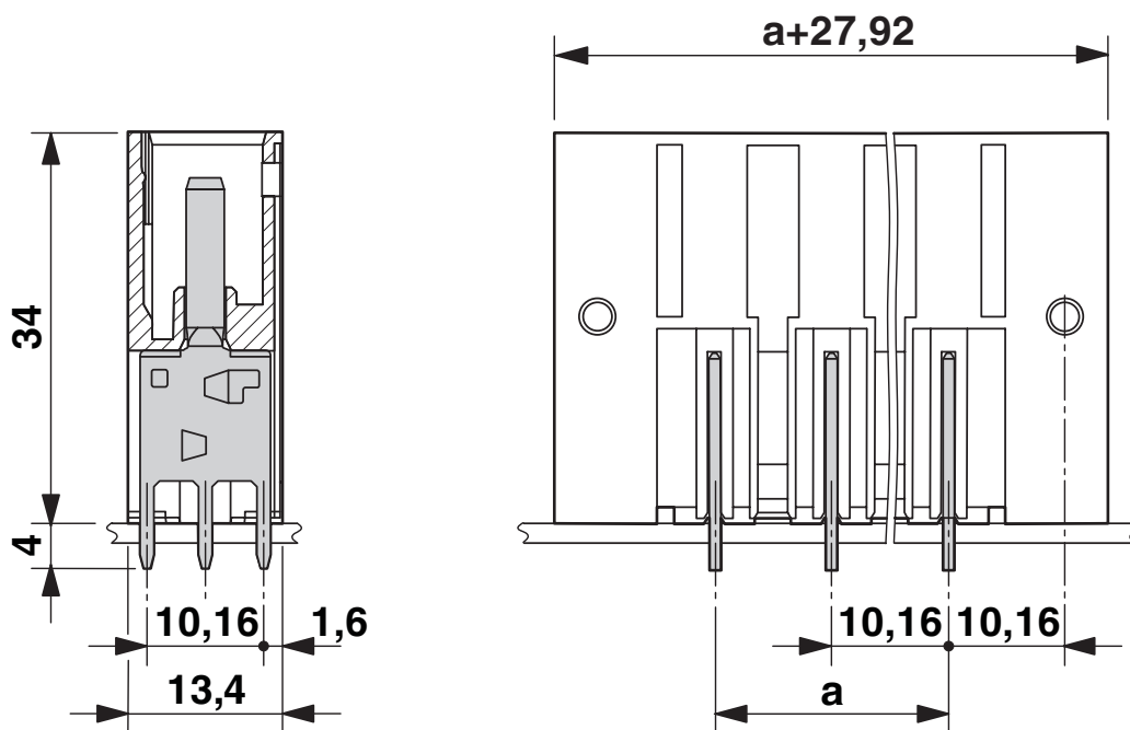
Maatschets
