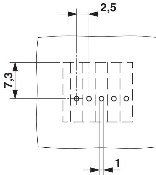
boorsjabloon/soldeerpadgeometrie
