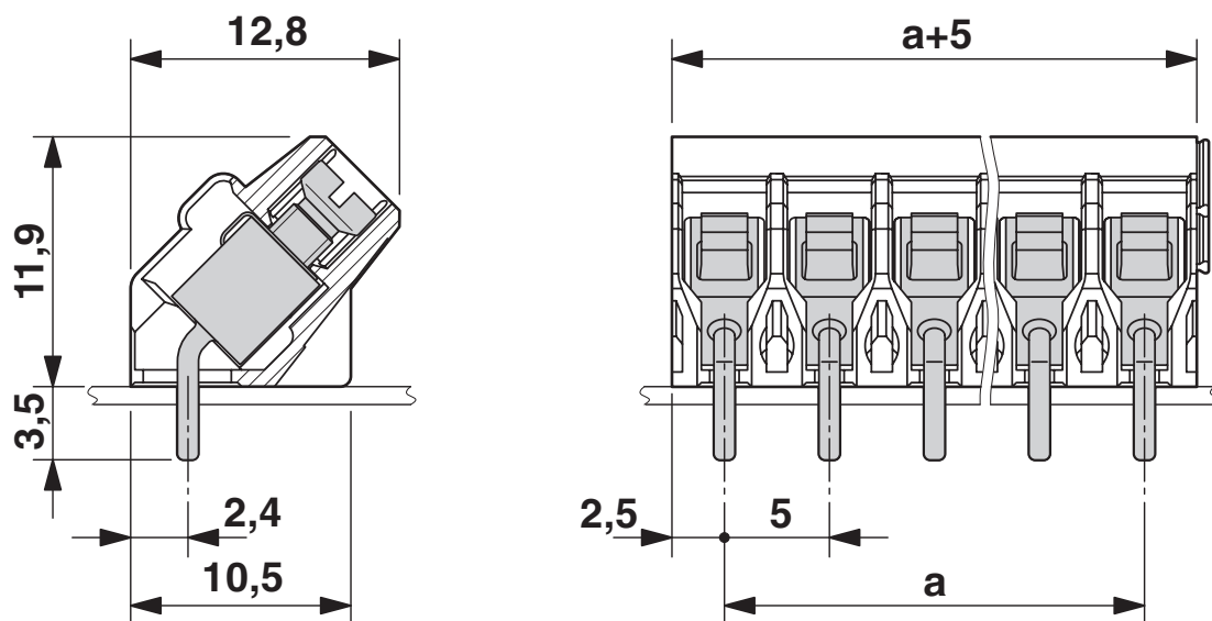
Maatschets
