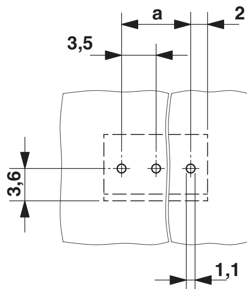
boorsjabloon/soldeerpadgeometrie
