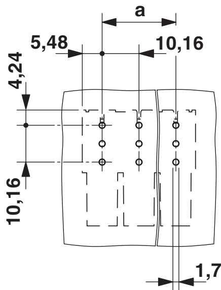
boorsjabloon/soldeerpadgeometrie
