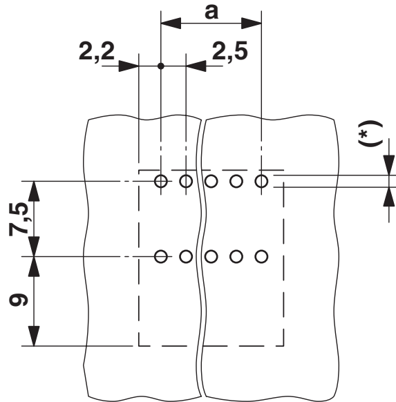
boorsjabloon/soldeerpadgeometrie
