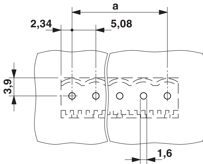
boorsjabloon/soldeerpadgeometrie
