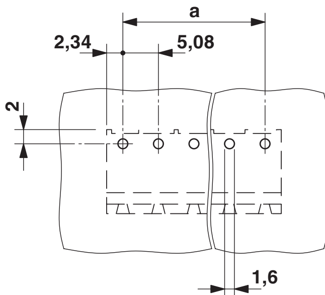
boorsjabloon/soldeerpadgeometrie
