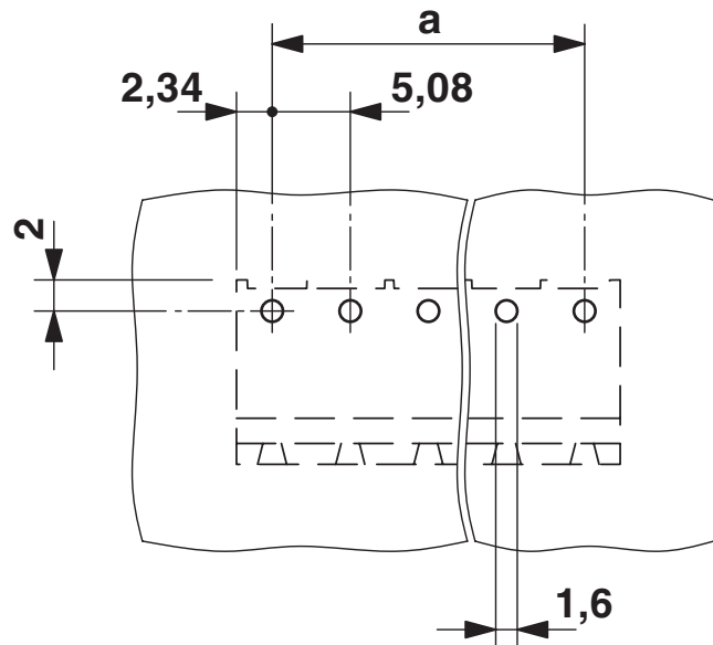
boorsjabloon/soldeerpadgeometrie
