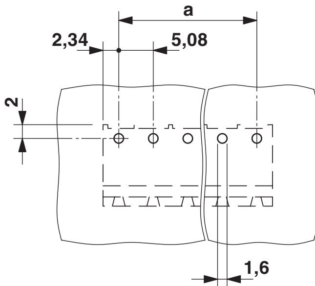
boorsjabloon/soldeerpadgeometrie
