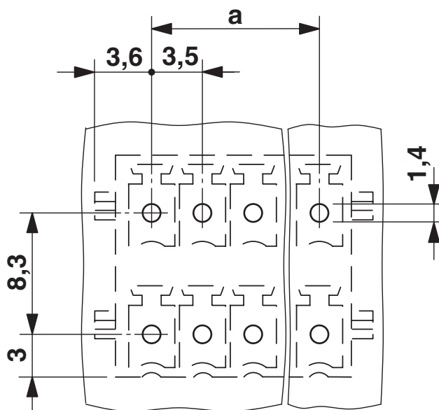
boorsjabloon/soldeerpadgeometrie
