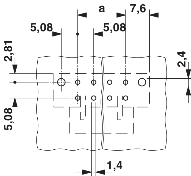
boorsjabloon/soldeerpadgeometrie
