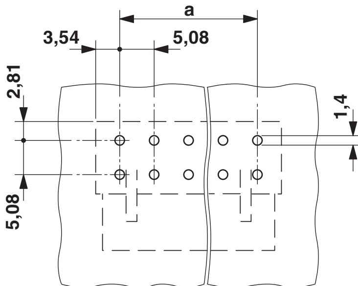
boorsjabloon/soldeerpadgeometrie
