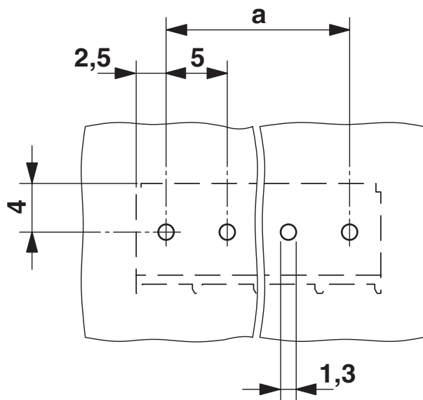
boorsjabloon/soldeerpadgeometrie
