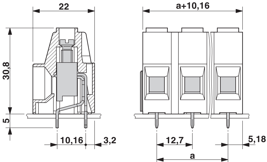
Maatschets
