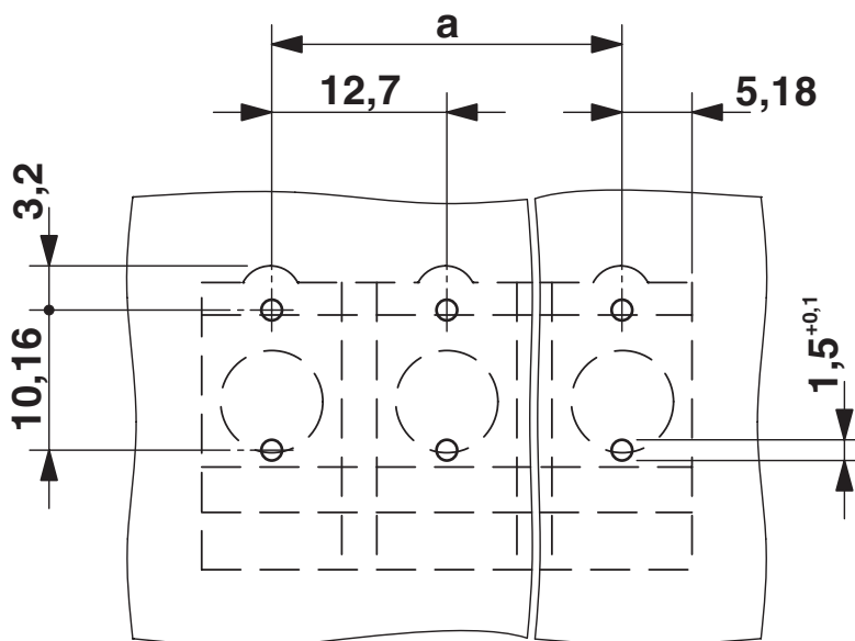
boorsjabloon/soldeerpadgeometrie
