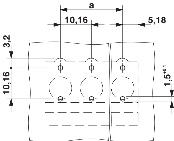
boorsjabloon/soldeerpadgeometrie
