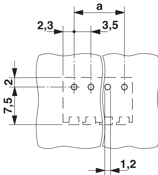
boorsjabloon/soldeerpadgeometrie
