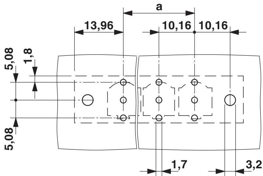
boorsjabloon/soldeerpadgeometrie
