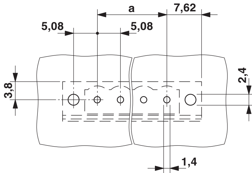
boorsjabloon/soldeerpadgeometrie
