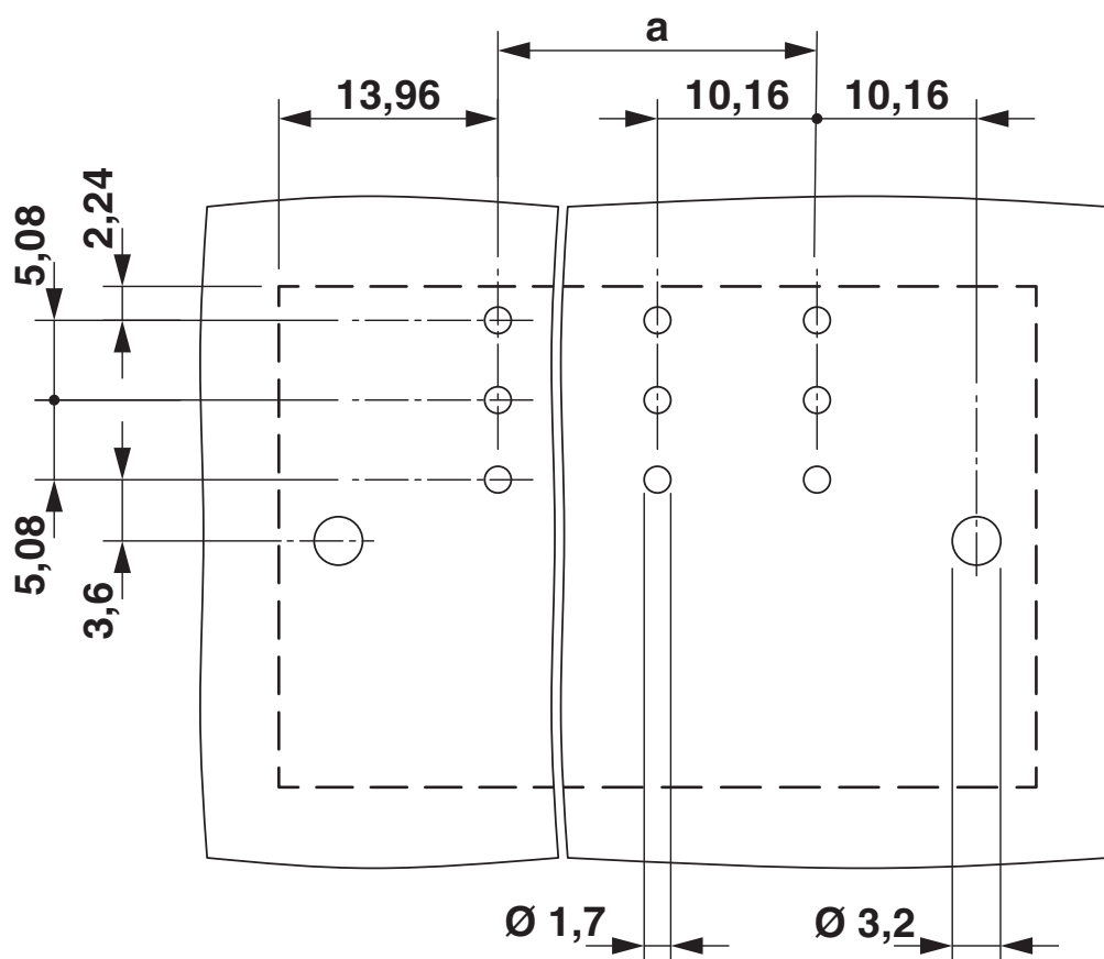
boorsjabloon/soldeerpadgeometrie
