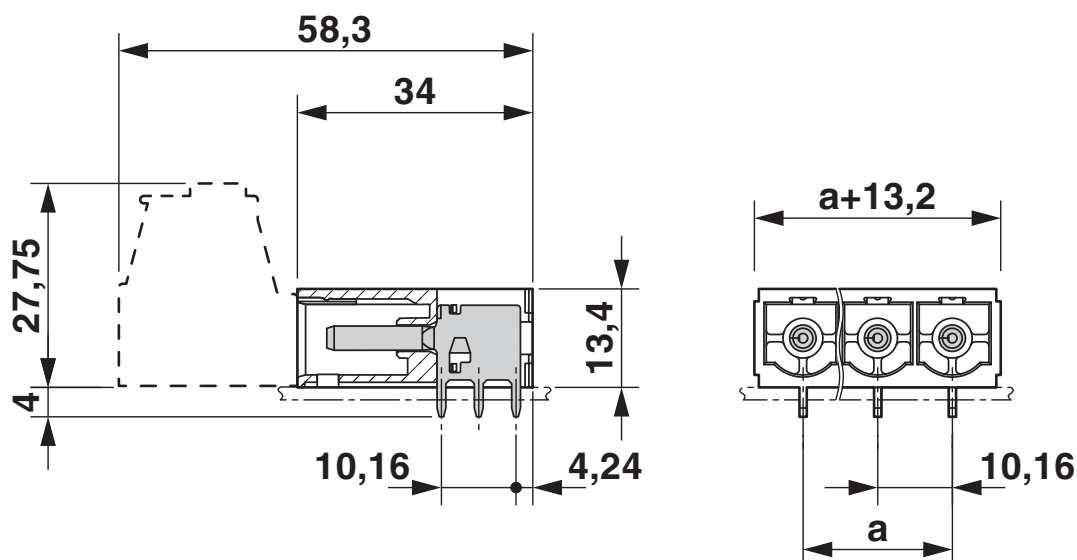
Maatschets
