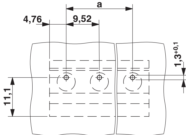
boorsjabloon/soldeerpadgeometrie
