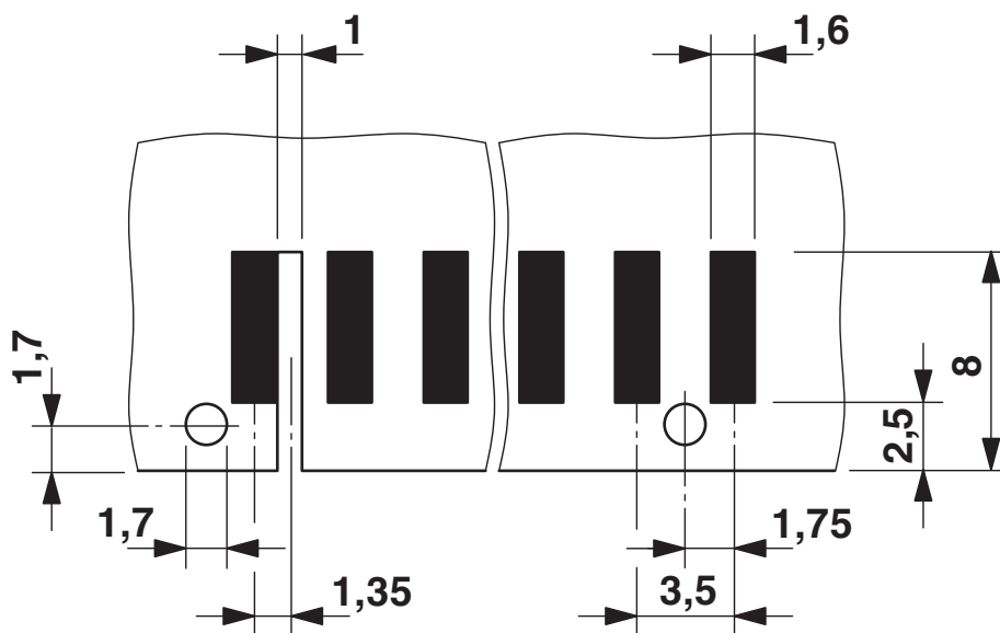
boorsjabloon/soldeerpadgeometrie
