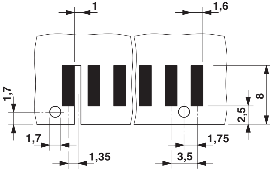
boorsjabloon/soldeerpadgeometrie
