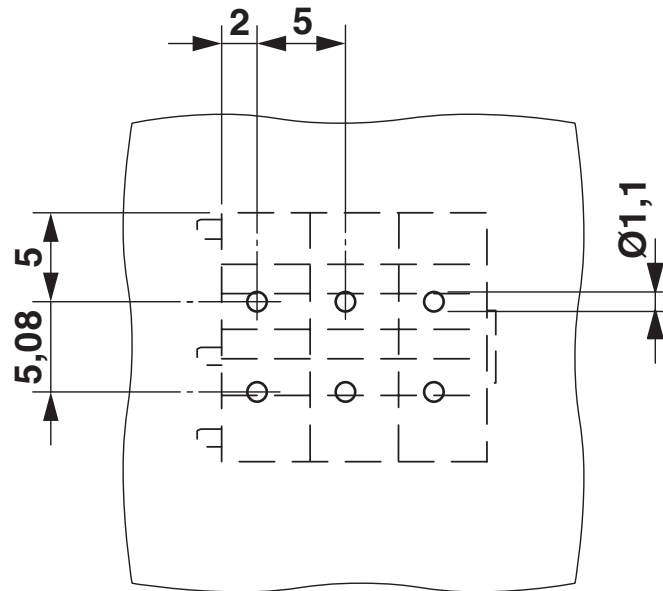
boorsjabloon/soldeerpadgeometrie
