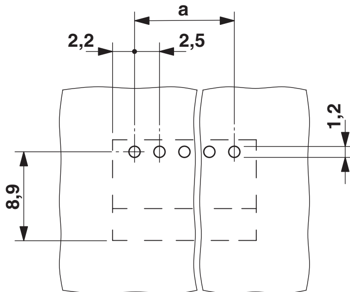
boorsjabloon/soldeerpadgeometrie
