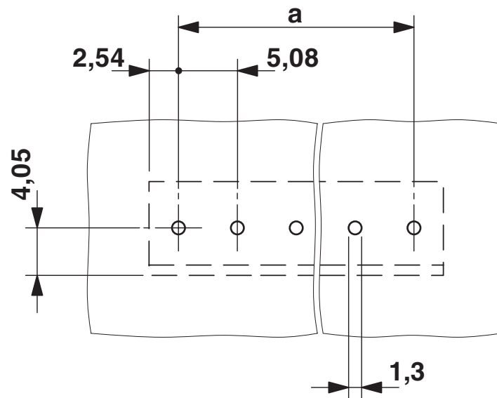
boorsjabloon/soldeerpadgeometrie
