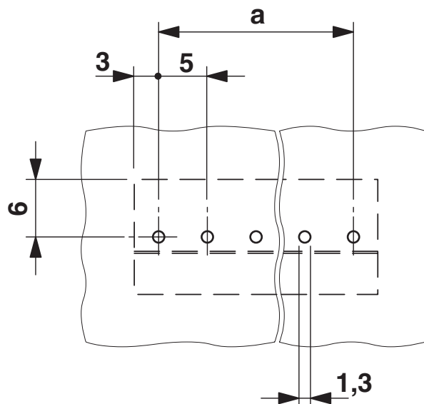
boorsjabloon/soldeerpadgeometrie
