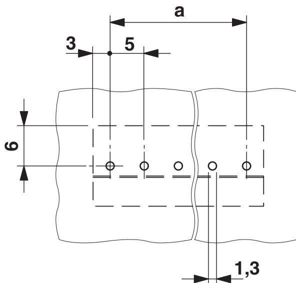
boorsjabloon/soldeerpadgeometrie
